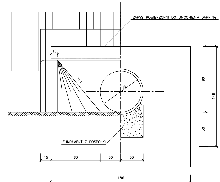
WIDOK OD STRONY WYLOTU PRZEKRÓJ 1-1
